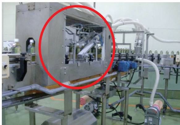
水切り装置のブロアー化（第3プラント）
