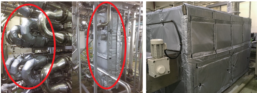
放熱ロス対策（タニガワプラント）左から、チューブU字配管、パストライザー放熱ロス対策（第1プラント）抽出温水 PL
